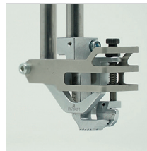
Felling feet Knappnahtfüße
