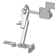
Combined roller and straight guide from the left Kombinierter Rollen- und Geradanschlag von links
