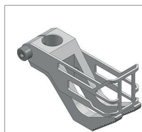
Sewing feet for triple feed machines for heavy-duty applications Nähfüße für Dreifachtransportmaschinen für schwere Anwendungen
