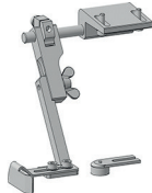
Reinforced combined roller and straight guide, from the right Verstärkter kombinierter Rollen- und Geradanschlag von rechts
