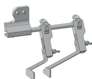
Two piece edge guide from the right Zweiteiliger Kantenanschlag von rechts
