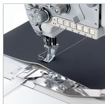
Assembly kit for listing tape guide Teilesatz Schlauchbandführung
