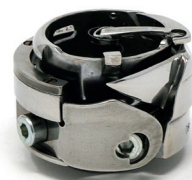
Hook 26 mm Ø Short thread trimmer Completed assembly - 0867 150914 Greifer 26 mm Ø Kurzfasenabschneider Gesamte Baugruppe - 0867 150914
